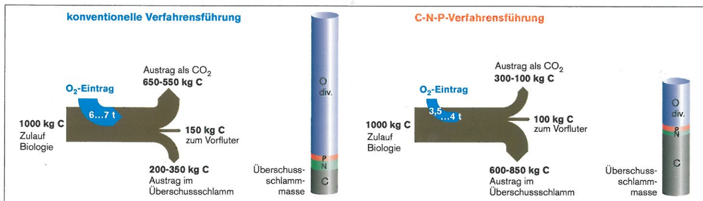
DAS C-N-P-VERFAHREN: Kohlenstoffbilanz und Überschussschlamm-Masse
